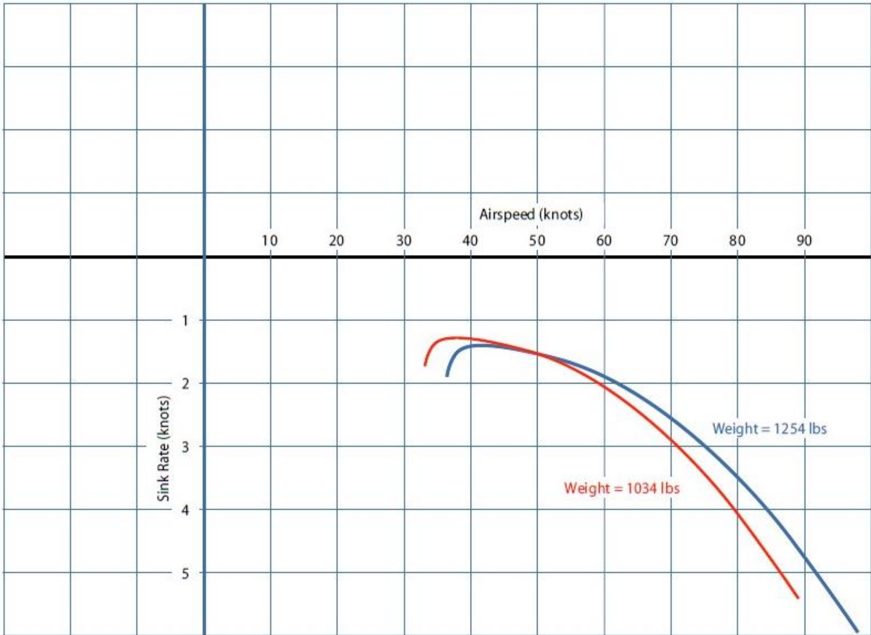
ASK-21 Polar
